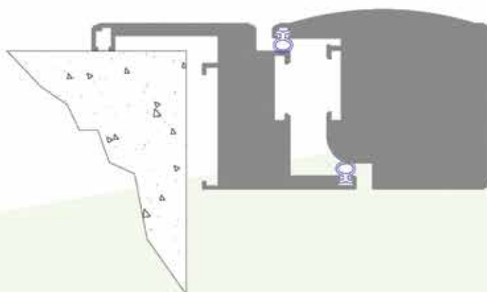
DETTAGLIO GEOMETRICO
