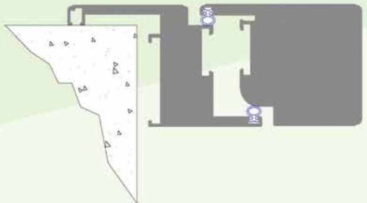
DETTAGLIO GEOMETRICO
