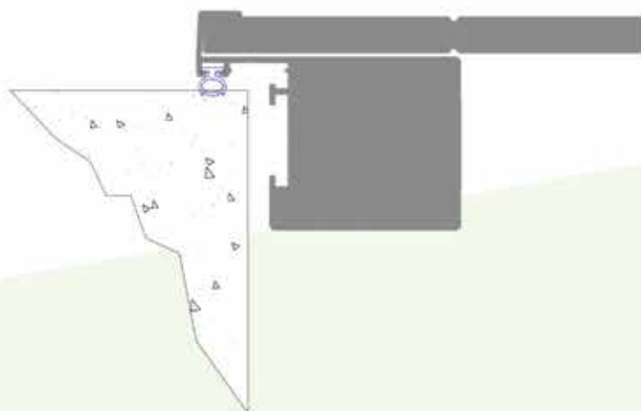
DETTAGLIO GEOMETRICO
