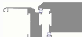
DETTAGLIO GEOMETRICO
