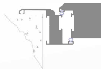
DETTAGLIO GEOMETRICO
